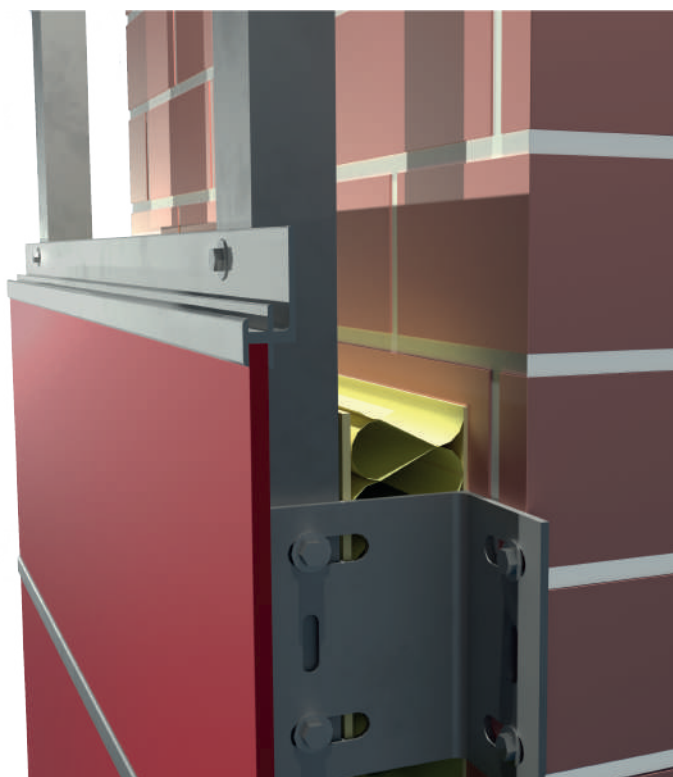
Anclajes en estructuras metálicas
