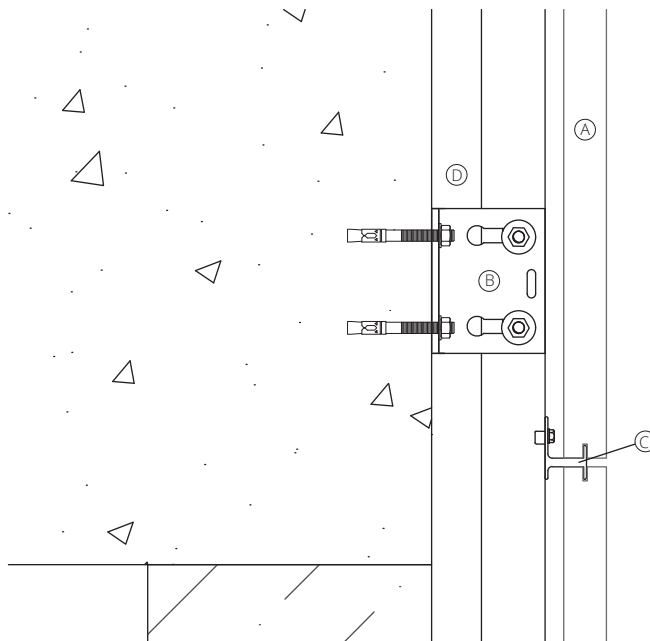
Anclaje Intermedio
