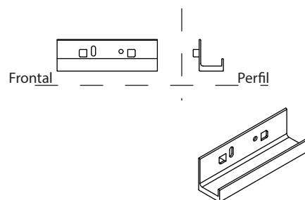
Anclaje Arranque - Terminación
