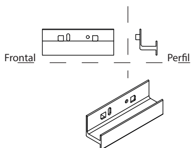
Anclaje Intermedio
